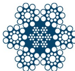
6x19 (9/9/1) IWRC
